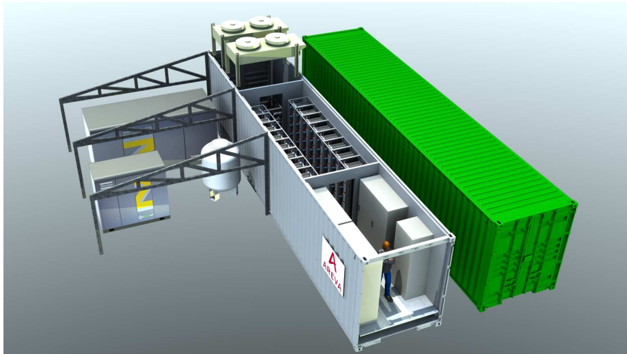
AREVA Stockage d'Énergie - Concept d'une pile à combustible de 2MW
